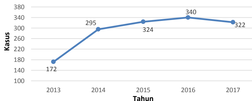
Grafik 3.14 Angka Kecelakaan Lalu Lintas Tahun 2013-2017
